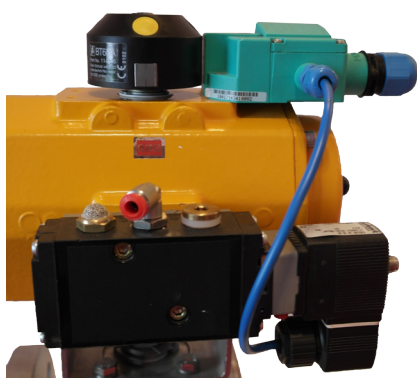
Pneumatische bediening met eindeloopschakelaar doorverbonden met magneetventiel
